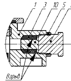
ж) монтаж заглушки ЗГ
