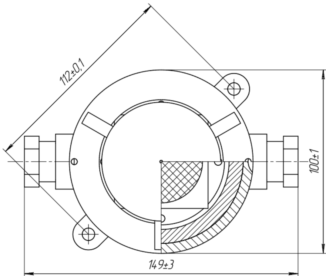
1 – монтажная плата; 2 - БИЗ; 4 - корпус; 5 - вставка; 6 - крышка; 7 – защитная сетка; 8 – прокладка; 9 – кабельный ввод; 10 – кольцо уплотнительное; 25 – дымовая камера.
