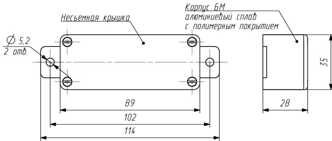
Рисунок Е.1 – Блок магнитов БМ1а – штатный блок магнитов, или БМ2а – блок магнитов по заказу
